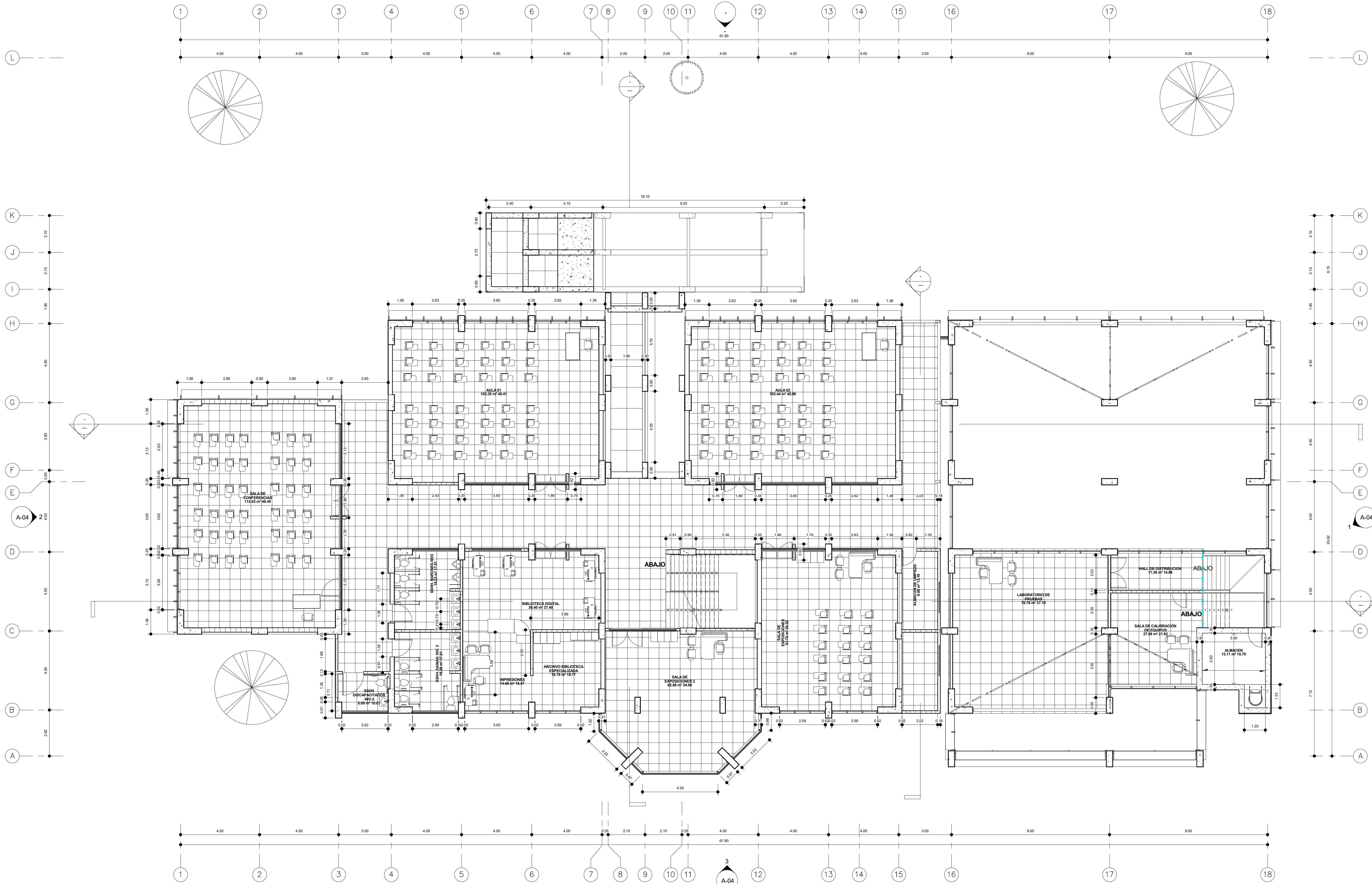
1 DISTRIBUCION NIVEL 02 1 : 100
