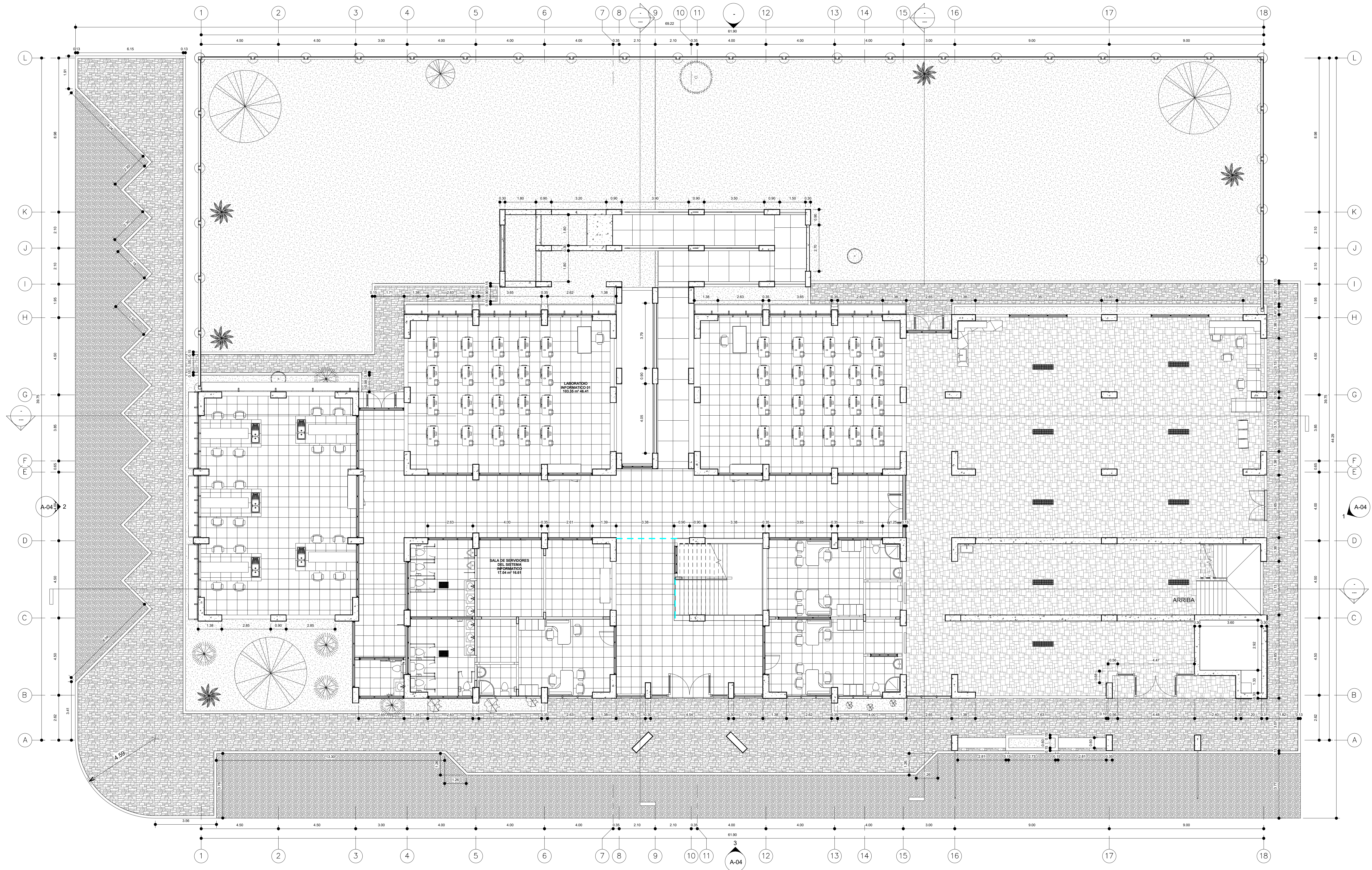
1 DISTRIBUCION NIVEL 01 1 : 100
